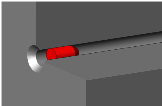
Rys. 4. Montaż korka Swell Sil w rurce dystansowej do ściągą
